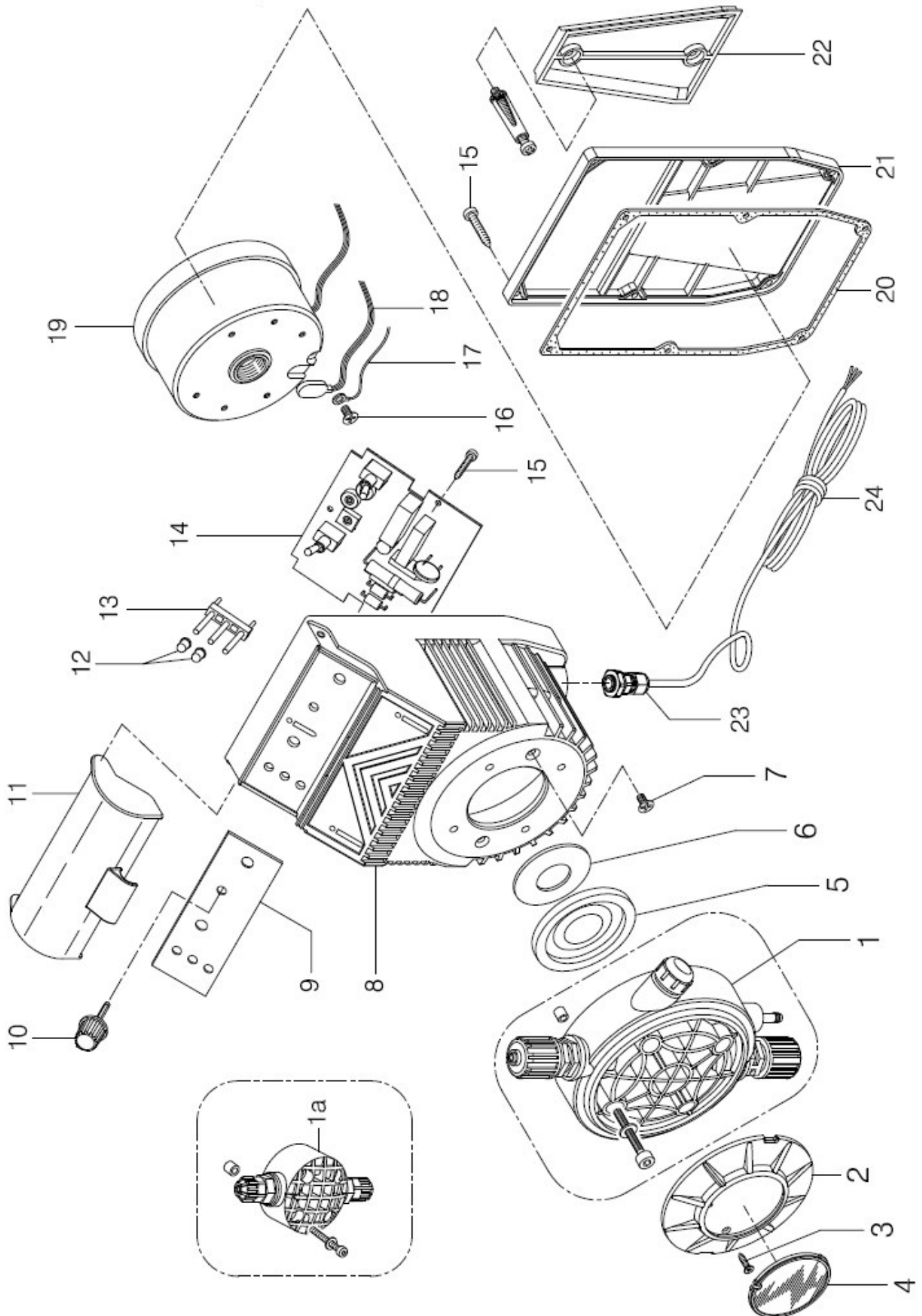
Fig. 10 SERIE EC 100 - Esploso / Description / Explode / Dibujo
